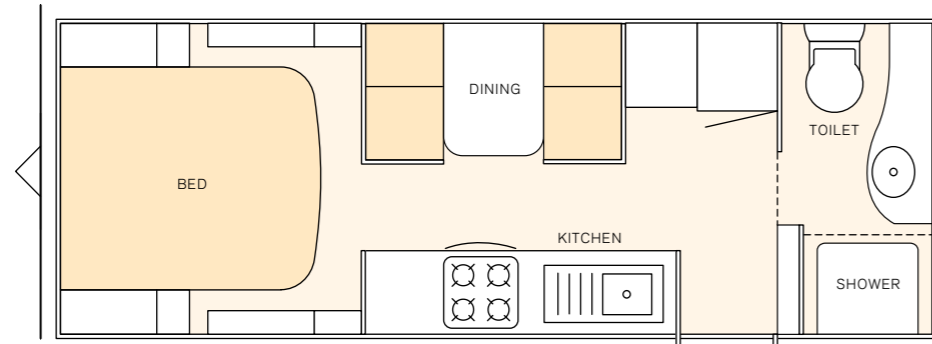
OZ CLASSIC 20FT (OZ20ES4)
